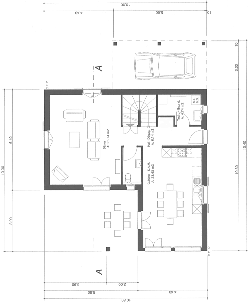
MODEL 5.0 - Rez-de-chaussée
