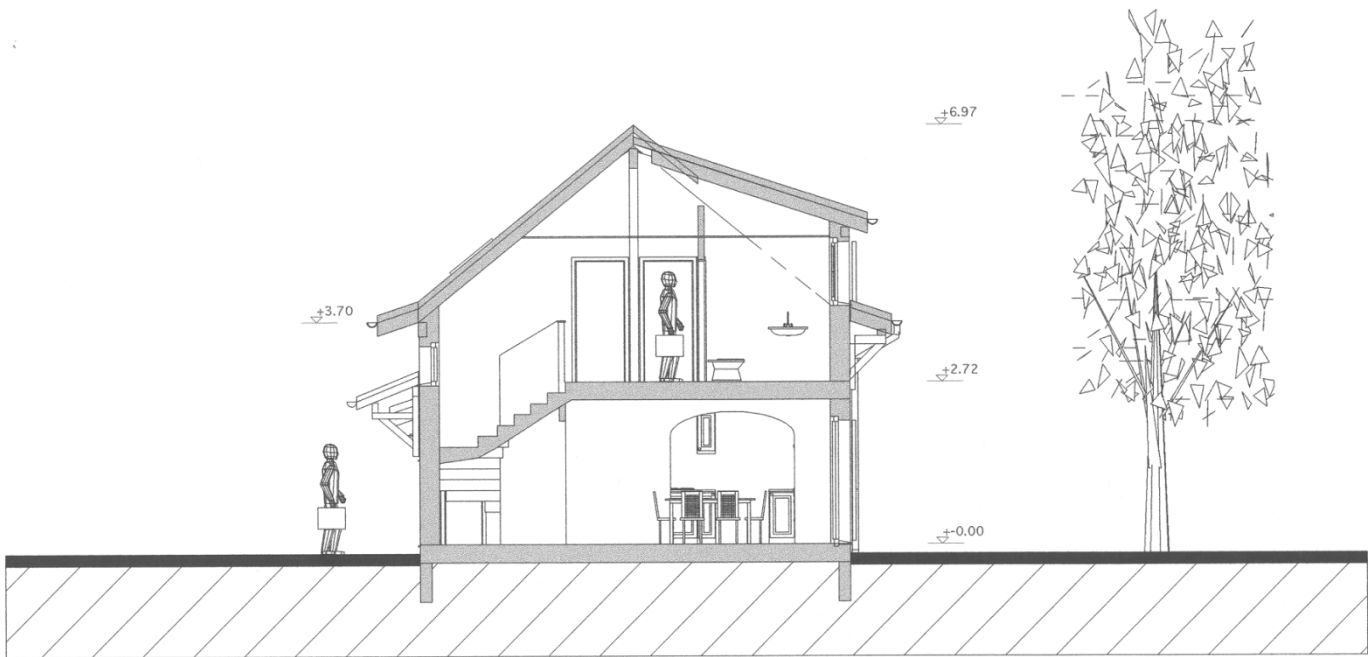
MODEL 2.9 - Coupe A-A
